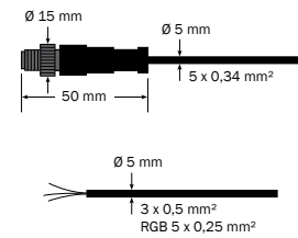
Einbautiefe mit Gehäusestecker + 60 mm Installation depth with housing plug + 60 mm Profondeur d'encastrement avec la fiche du boîtier + 60 mm
